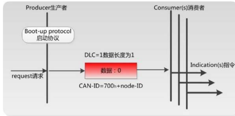
图 2-2 节点上线报文
