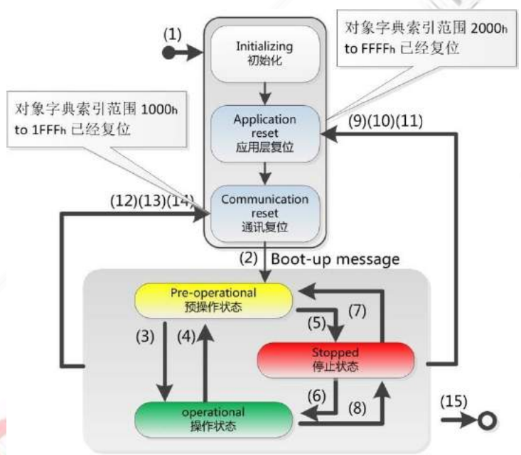
图 2-1 NMT 管理状态转换图
