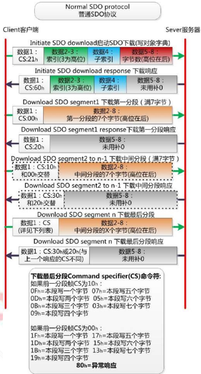
图 2-9 普通 SDO 下载协议
